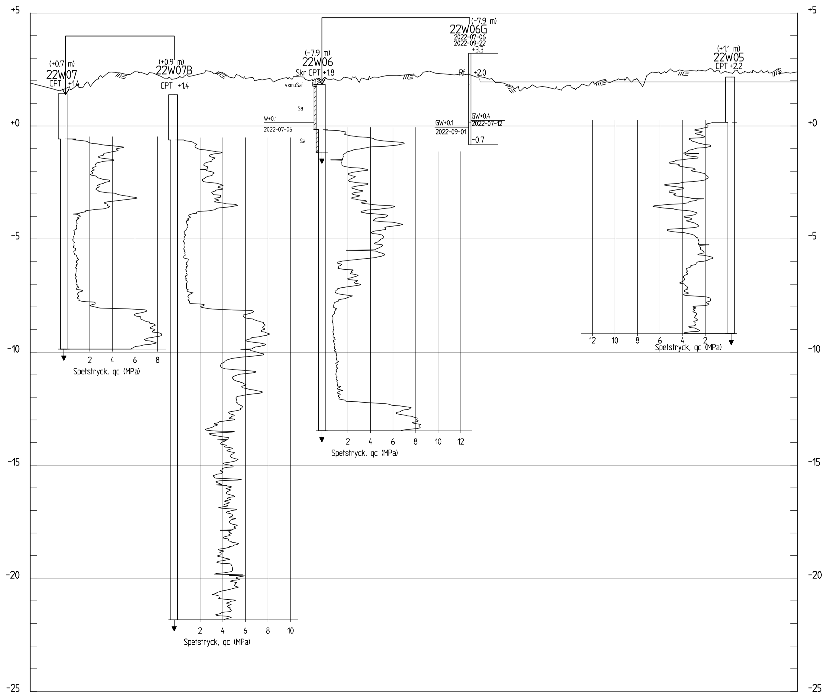
SEKTION D-D H 1:100 L 1:500
