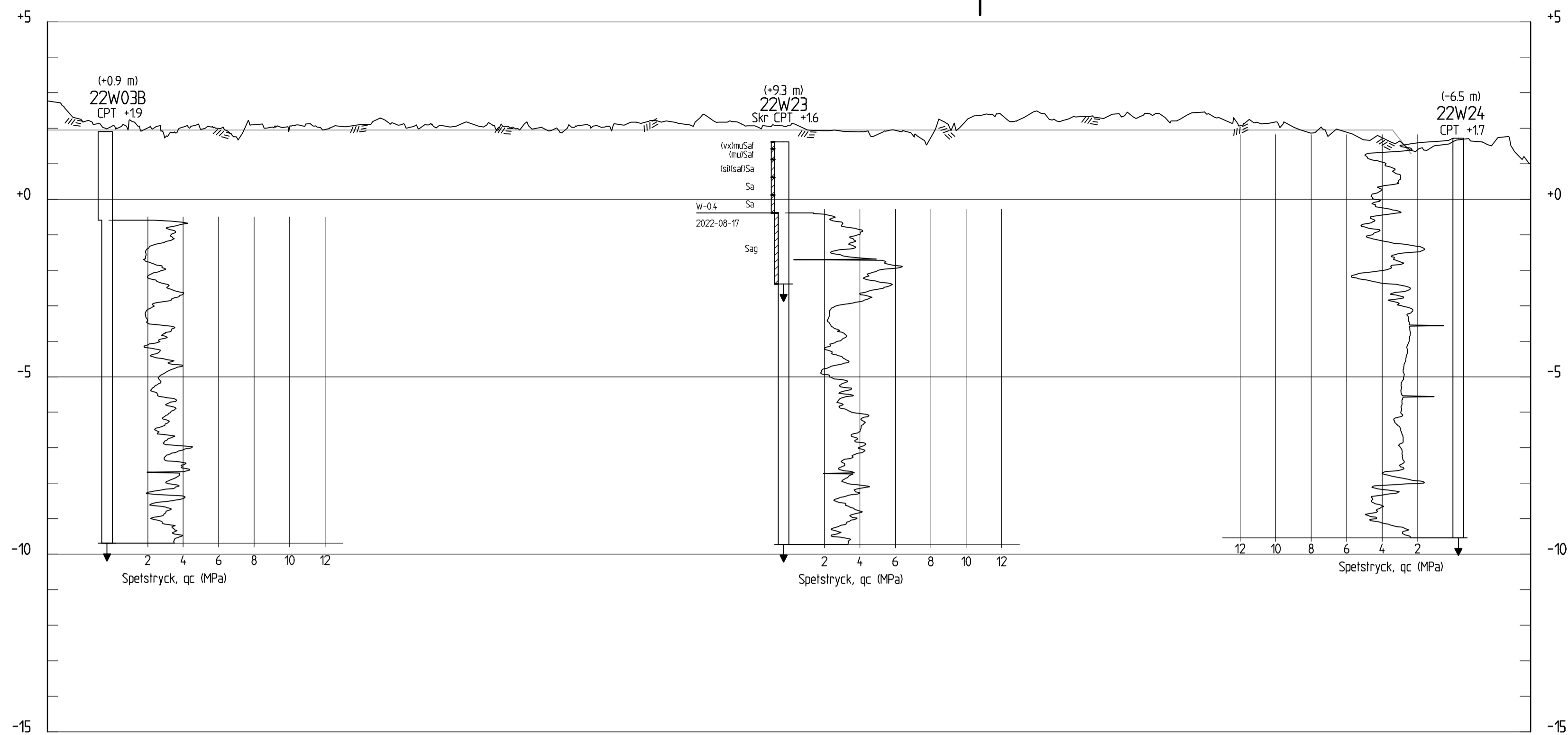
SEKTION C-C H 1:100 L 1:500
